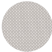
Pumice
